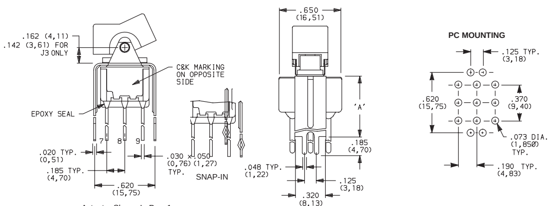
7301J1_BE2 3PDT
