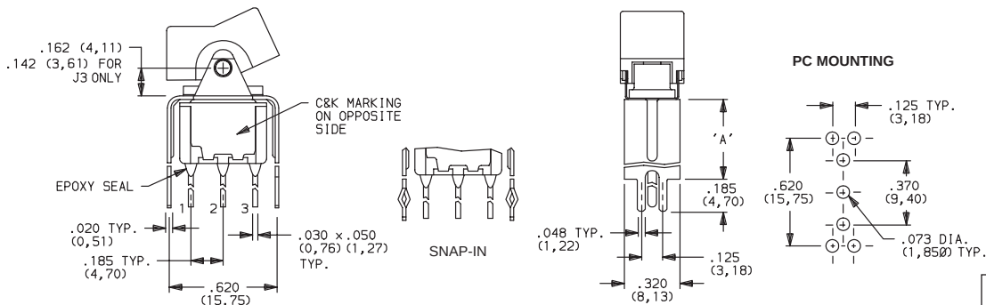
7101J1_BE2 SPDT
