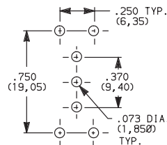
7101J1_BE2 SPDT
