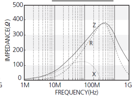
CIM03U241
