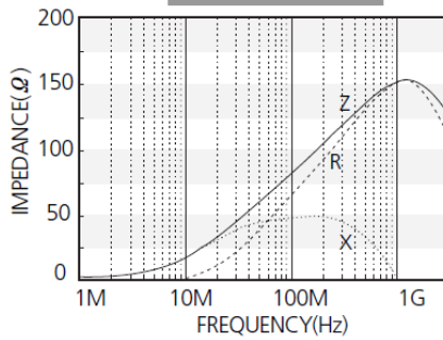
CIM03U800
