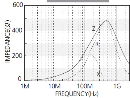
CIM03J241
