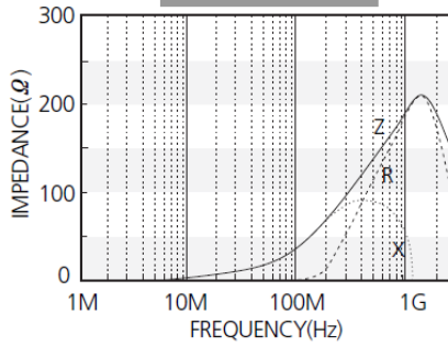
CIM03U800
