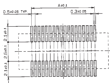
基板取付け寸法 MOUNTING LAYOUT
