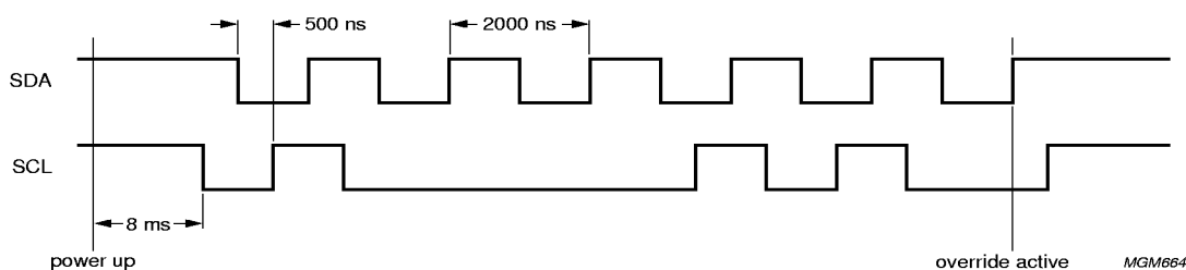
Fig.3 POR override sequence.
