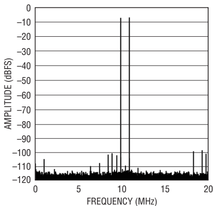
LTC2181: 64k Point 2-Tone FFT, f_{IN} = 69\text{MHz} , 70\text{MHz} , -7\text{dBFS} , 40\text{Mps}
