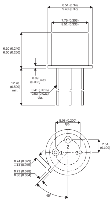
TO39 (TO205AD)
