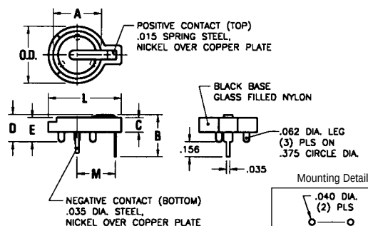
DWG. 2
