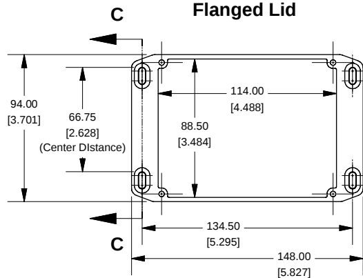
Flanged Lid
