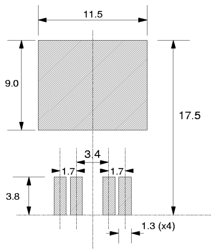
Fig.39. SOT426
