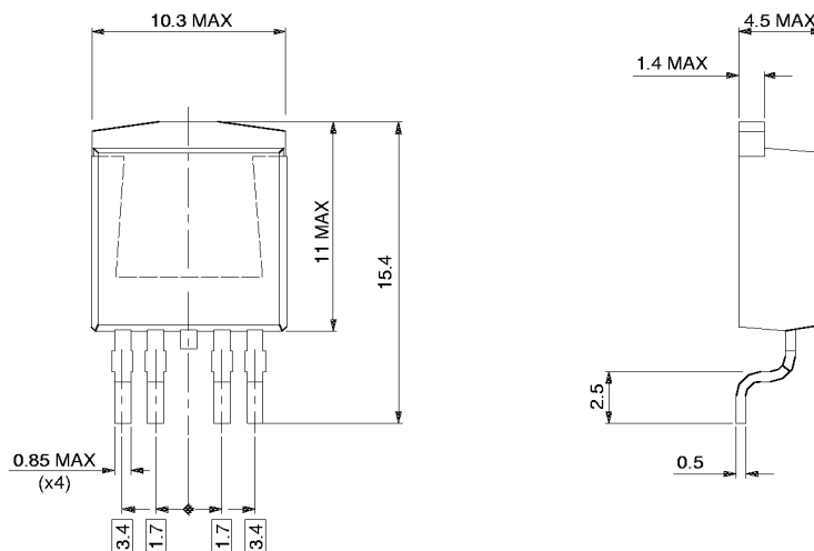
Fig.38. SOT426
