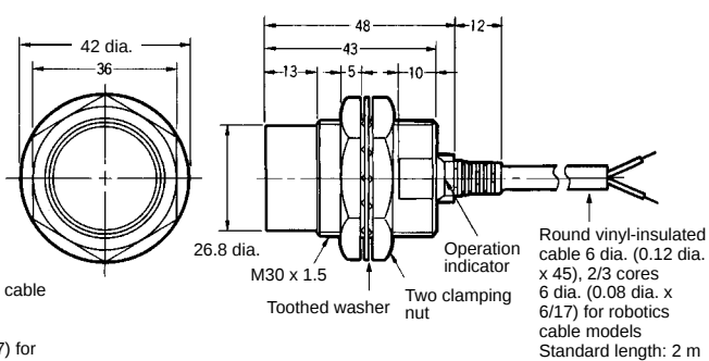
Fig. 16 : E2E-X20MD□/E2E-X18ME□/F□ E2E-X18MY□
