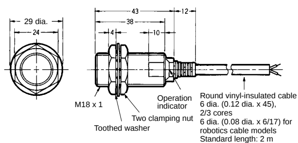
Fig. 15 : E2E-X10D□-N/E2E-X10E□/F□ E2E-X10Y□/E2E-X10T1
