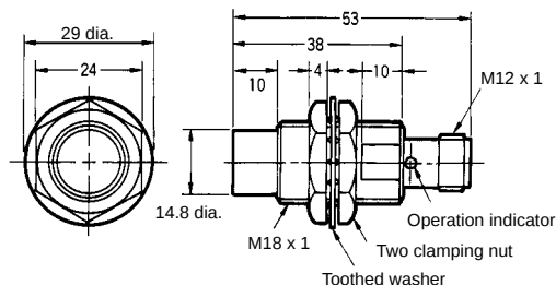
Fig. 26 : E2E-X20MD□-M1G/E2E-X18ME□-M1/F□-M1 E2E-X18MY□-M1
