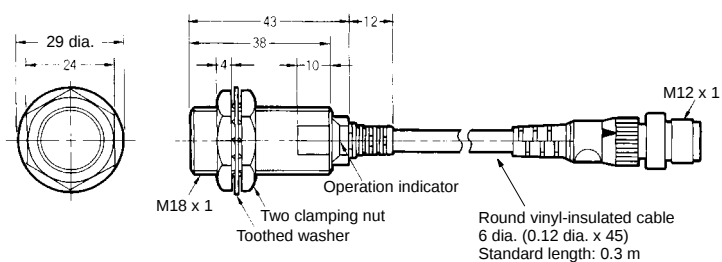
Fig. 31 : E2E-X7D1-M1GJ E2E-X7D1-M1J-T
