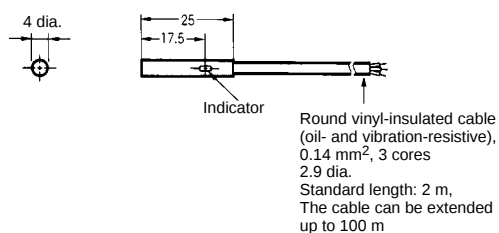
Fig. 3 : E2E-C1□□
