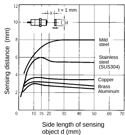
E2E-X1R5E□/F□
