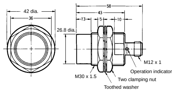
Fig. 26 : E2E-X20MD□-M1G/E2E-X18ME□-M1/F□-M1 E2E-X18MY□-M1
