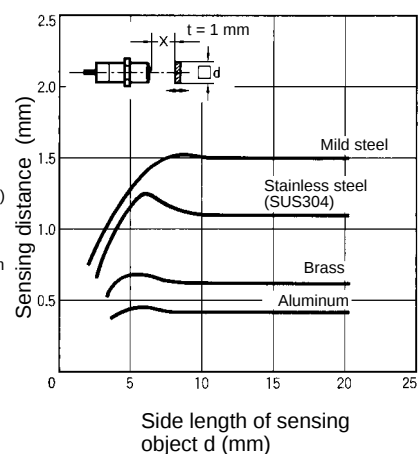
E2E-X1R5Y□
