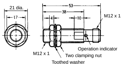
Fig. 23 : E2E-X7D□-M1G/E2E-X5E□-M1/F□-M1 E2E-X5Y1-M1
