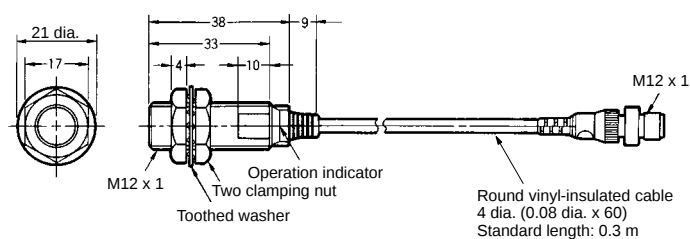
Fig. 30 : E2E-X8MD1-M1GJ
