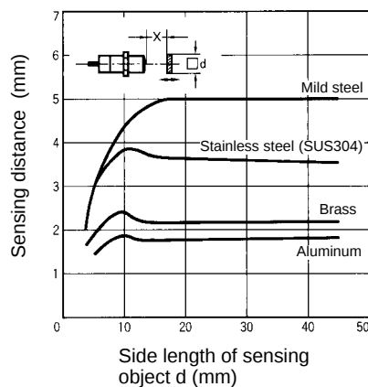
E2E2-X5MC□/B□ E2E2-X5MY□
