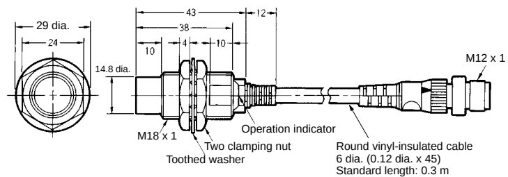
Fig. 33 : E2E-X10D1-M1GJ E2E-X10D1-M1J-T
