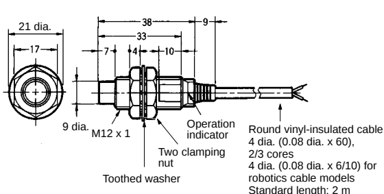
Fig. 9 : E2E-X8MD□ E2E-X5ME□/F□
