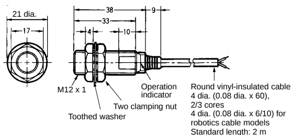
Fig. 8 : E2E-X3D□-N E2E-X2E□/F□
