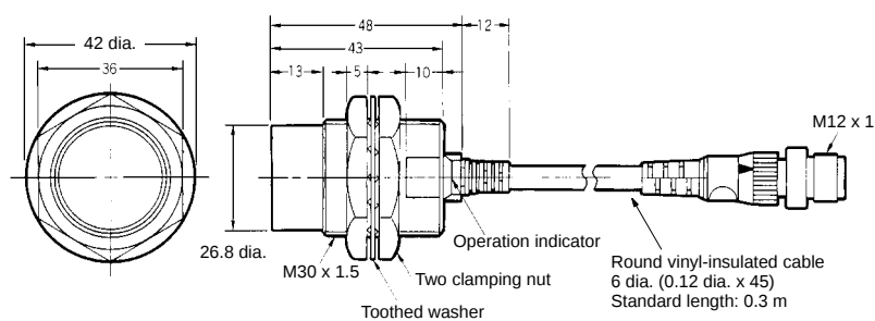
Fig. 34 : E2E-X20MD1-M1GJ
