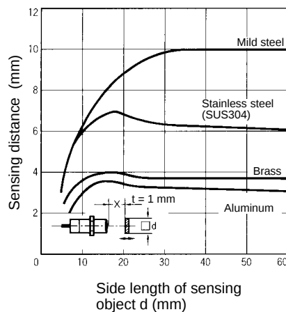
E2E-X10ME□/F□ E2E-X10MY□
