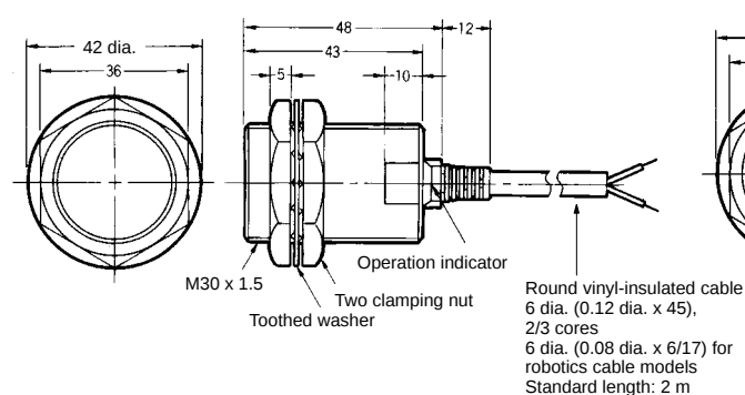
Fig. 15 : E2E-X10D□-N/E2E-X10E□/F□ E2E-X10Y□/E2E-X10T1
