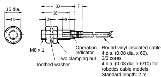
Fig. 6 : E2E-X1R5Y□
