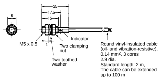
Fig. 2 : E2E-X1□□
