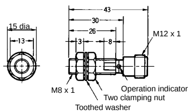
Fig. 19 : E2E-X3D□-M1G E2E-X2E□-M1/F□-M1
