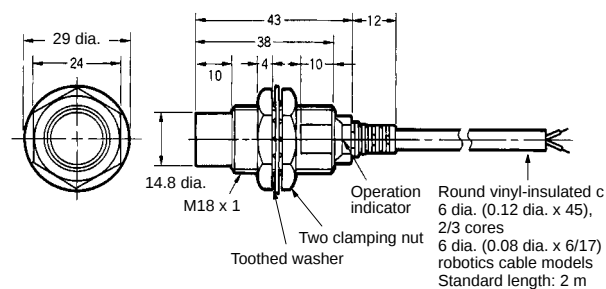
Fig. 16 : E2E-X20MD□/E2E-X18ME□/F□ E2E-X18MY□
