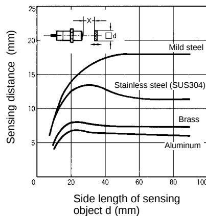
E2E2-X18MC□/B□ E2E2-X18MY□
