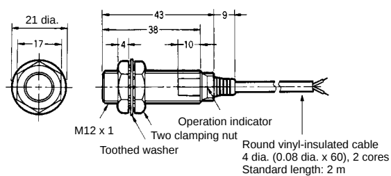
Fig. 10 : E2E-X2Y□
