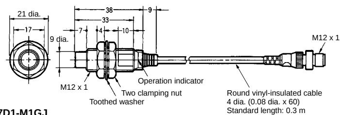
Fig. 31 : E2E-X7D1-M1GJ E2E-X7D1-M1J-T
