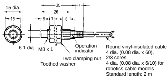
Fig. 5 : E2E-X4MD□ E2E-X2ME□/F□
