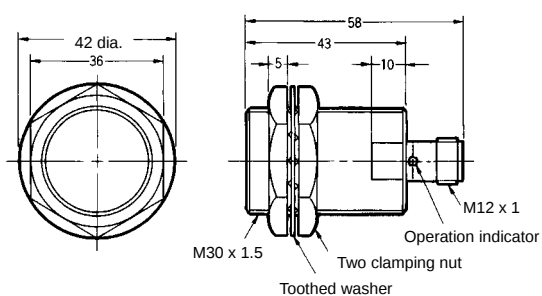
Fig. 25 : E2E-X10D□-M1G/E2E-X10E□-M1/F□-M1 E2E-X10Y1-M1
