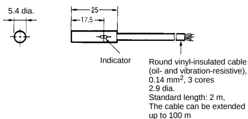
Fig. 3 : E2E-C1□□
