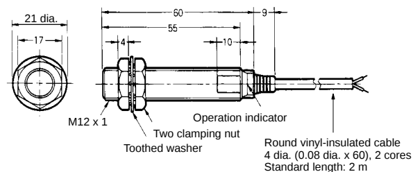
Fig. 13 : E2E-X7D□-N/E2E-X5E□/F□ E2E-X5Y□/E2E-X7T1
