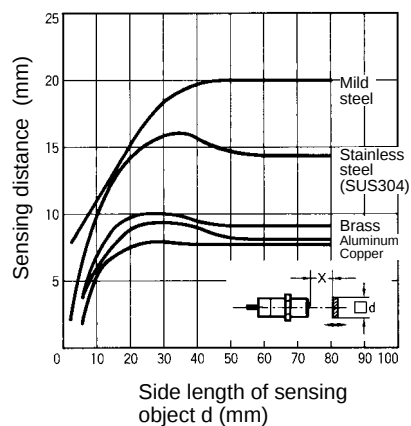
E2E2-X20MD□
