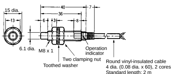
Fig. 9 : E2E-X8MD□ E2E-X5ME□/F□
