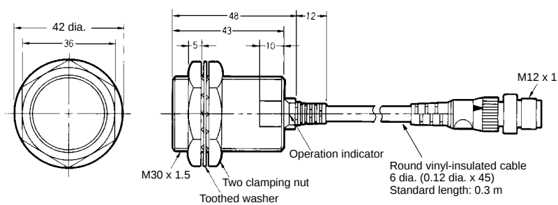
Fig. 34 : E2E-X20MD1-M1GJ
