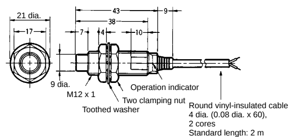
Fig. 11 : E2E-X5MY□
