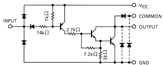
TD62387AP, TD62387AF
