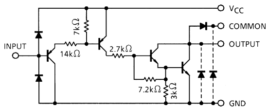
TD62388AP,TD62388AF
