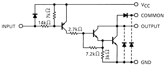
TD62388AP,TD62388AF
