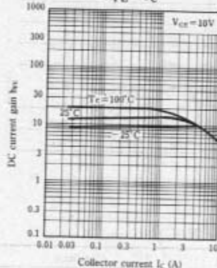
h_{FE} - I_C
