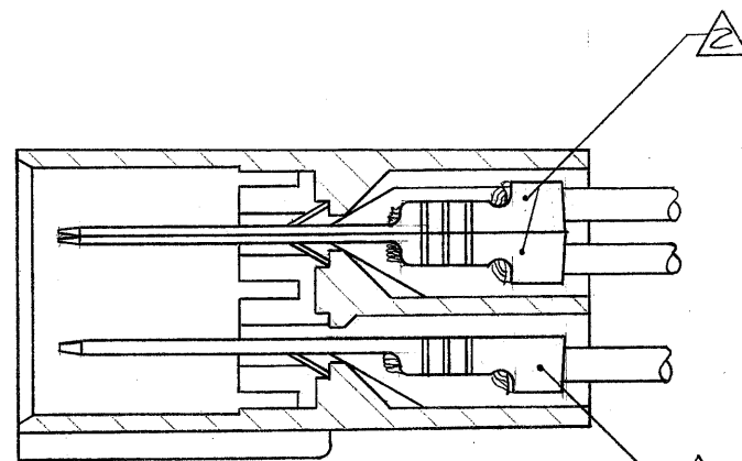
ファスティーファストンタブ接合状態 (FASTIN-FASTON TAB MATING STATE)
