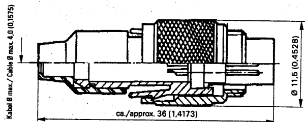
Maßzeichnung Drawing mm (inch)
