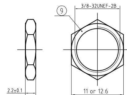
HEX NUT
