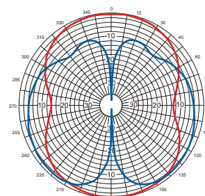
2.4 GHz — H-Plane — E-Plane
