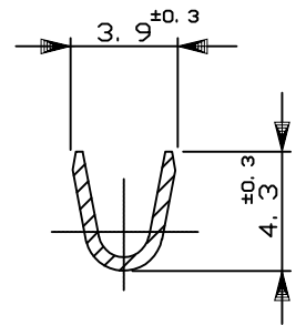
SECT. 断面 A-A
