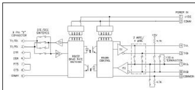
Blockdiagramm
