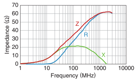
MPZ0603S330C
