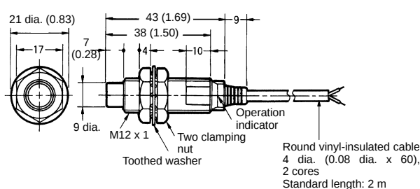
Fig. 6: E2E-X10MY□-N
