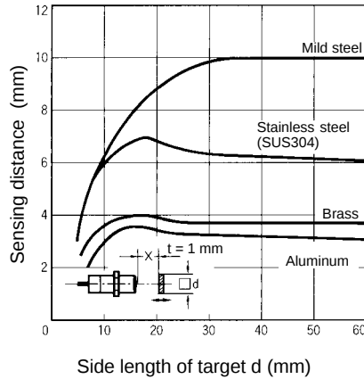
E2E-X10MY-N
