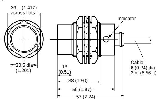
E2E-X18MY□-53-US
