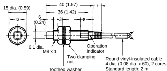
Fig. 2: E2E-X2MY□-N
