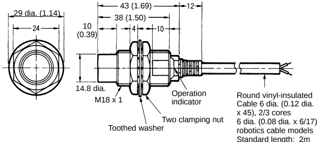
Fig. 6: E2E-X10MY□-N
