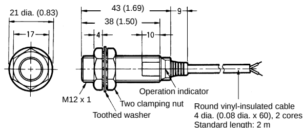
Fig. 3: E2E-X2Y□-N
