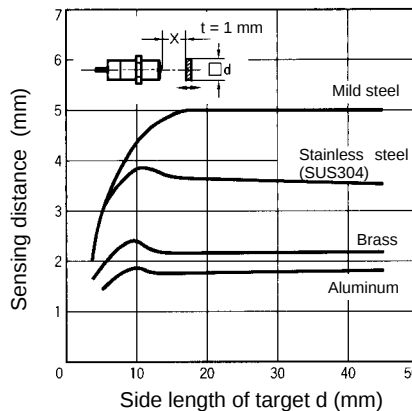
E2E-X5Y□-N
