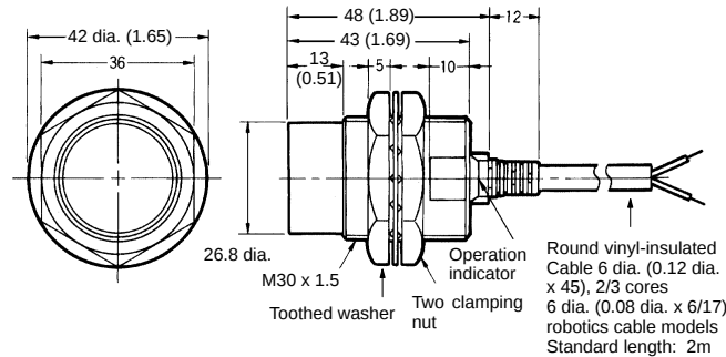
Fig. 8: E2E-X18MY□-N
