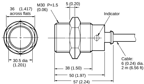
E2E-X10Y□-53-US
