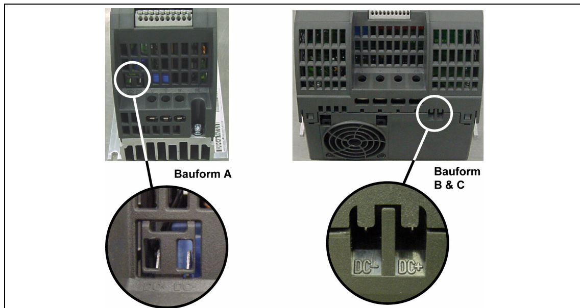
Bild 2-6 SINAMICS G110-DC-Anschlüsse
