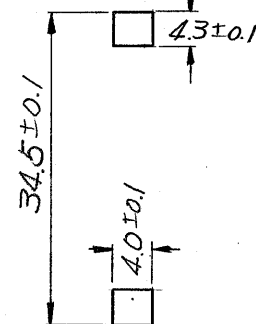
PANEL CUTTING DIMENSION パネル打抜寸法
