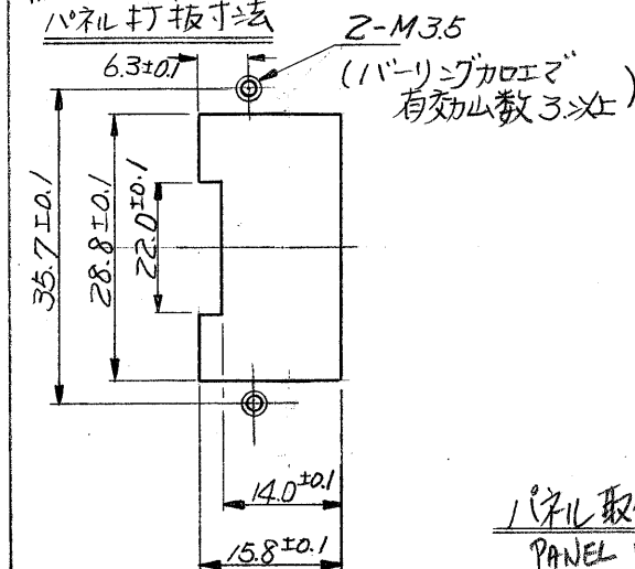
PANEL CUTTING DIMENSION パネル打抜寸法
