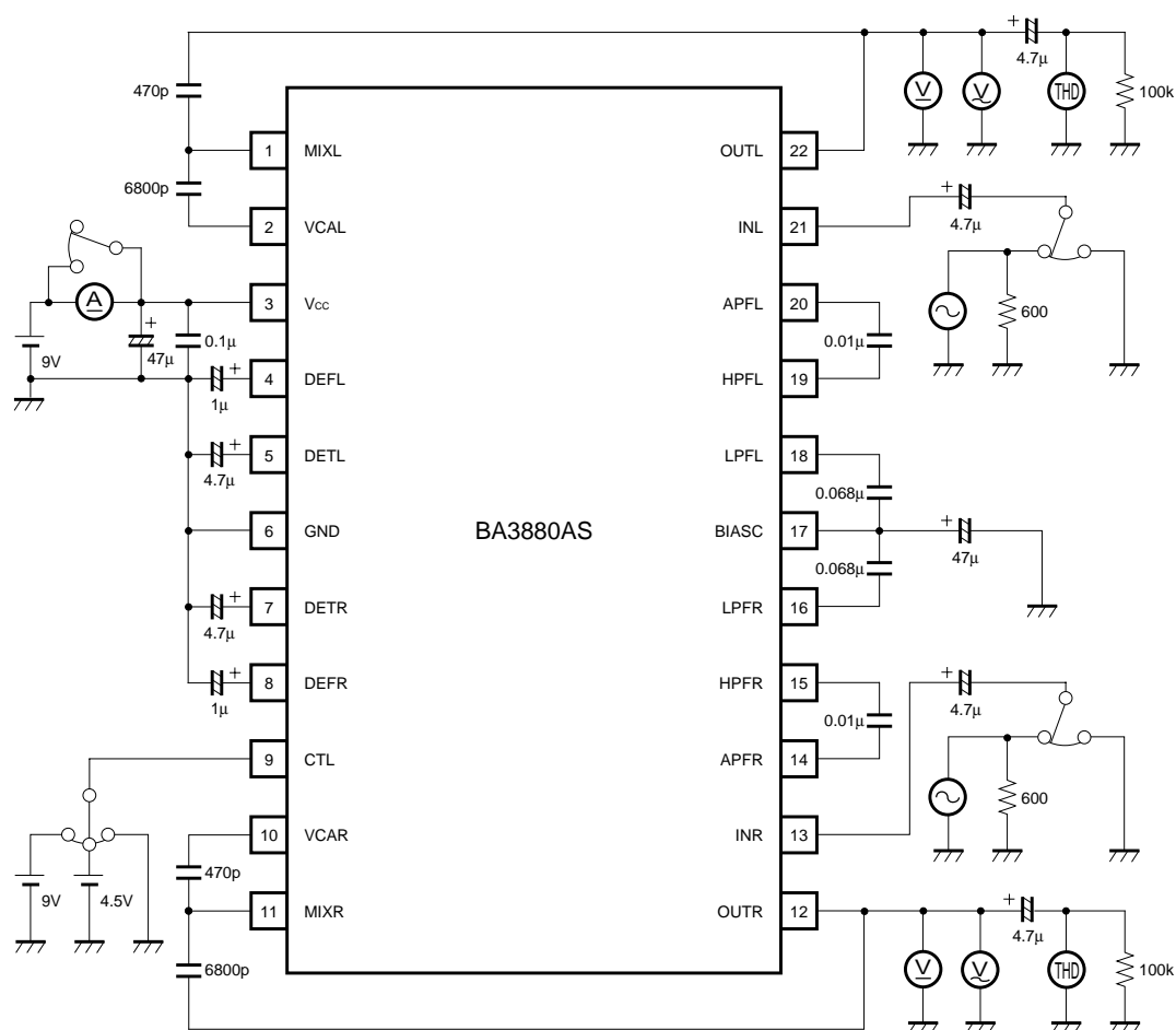
(Units) R : \Omega C : F
