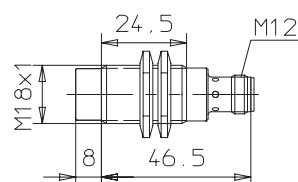
E2EL-X8M□-M1
