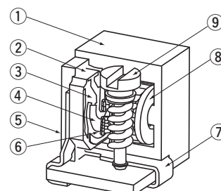
内部構造図 INTERNAL STRUCTURE
