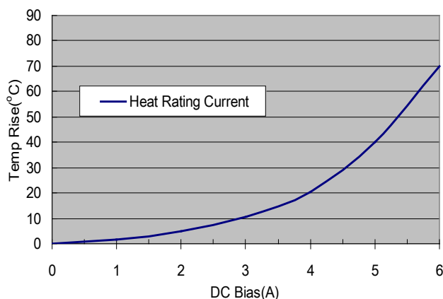
ASPI-0520LR-4R7
