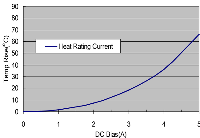
ASPI-0520LR-4R7
