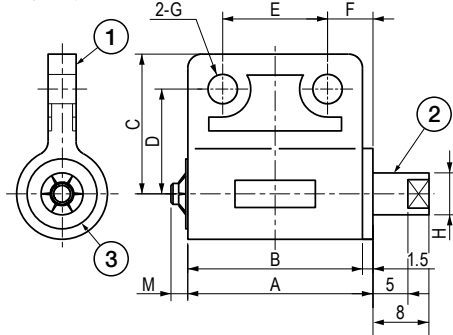
ヒンジ Hinge only
