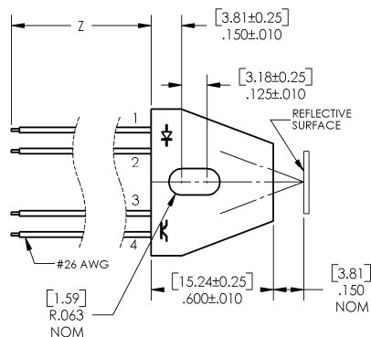
OPB746WZ, OPB747WZ,
