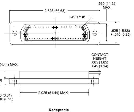
Receptacle
