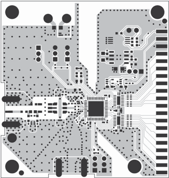
Top Side
