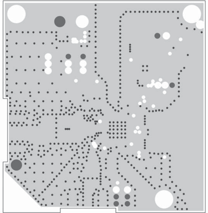
Inner Layer 3
