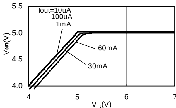
S-818A50A ( T_a=25^\circ\text{C} )
