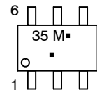
SOT-363 CASE 419B
