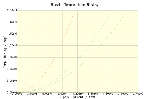
C2012X7R1E474K125AA(100kHz) C2012X7R1E474K125AA(500kHz) C2012X7R1E474K125AA(1MHz)
