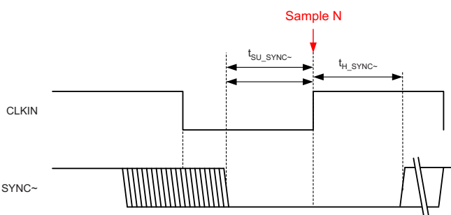
Figure 147. SYNC~ Timing (Subclass 2)
