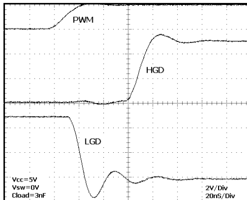
Fig 8. LGD Fall and HGD Rise Times
