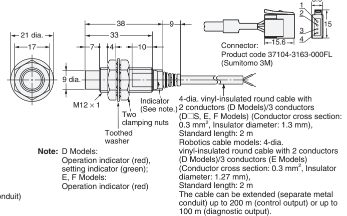
Fig. 10: E2E-X8MD□ E2E-X5ME□/F□
