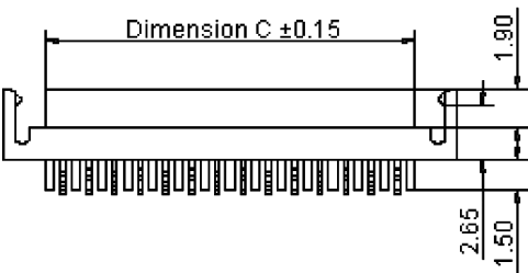
Dimensions : Millimetres
