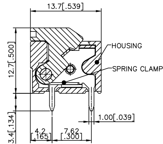
SEC. A-A
