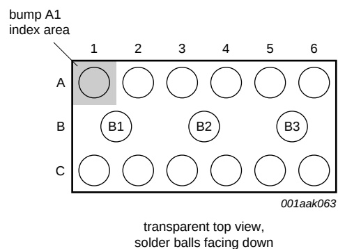
Fig 2. PEMI6CSP: pin configuration
