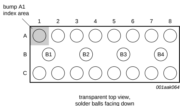
Fig 2. PEMI6CSP: pin configuration
