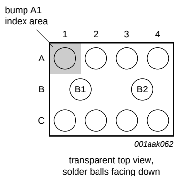
Fig 1. PEMI4CSP: pin configuration
