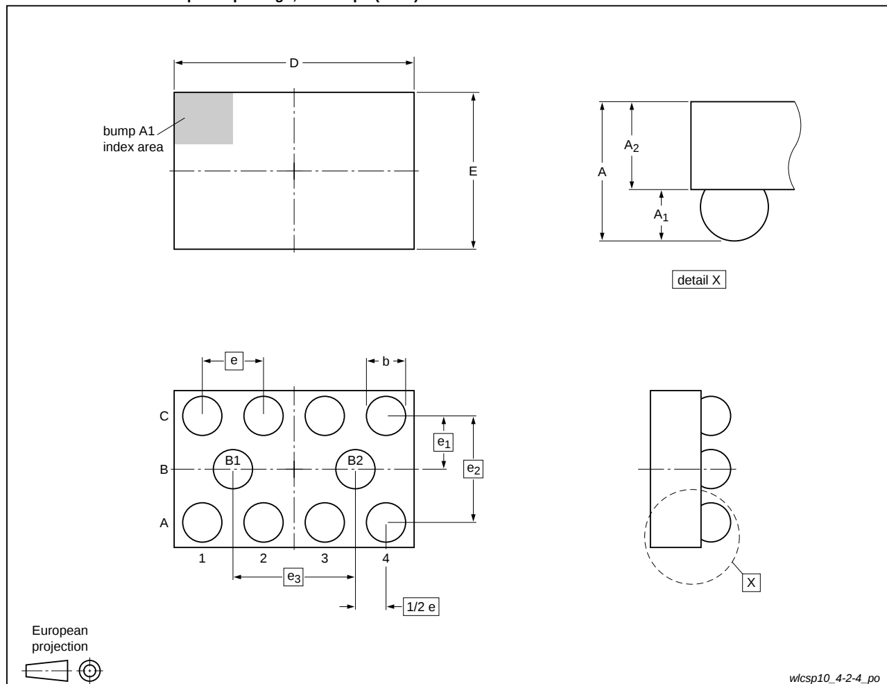
Fig 11. Package outline PEMI4CSP (WLCSP10)
