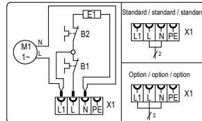
B1 Betriebsthermostat / Thermostat / Thermostat B2 Sicherheitsthermostat / Security thermostat / thermostat sécurité E1 Widerstandsheizung / Resistance Heater / Chauffage de résistance M1 Ventilator / fan / ventilateur X1 Klemmenkontakt / Connection mains / Contact tension
