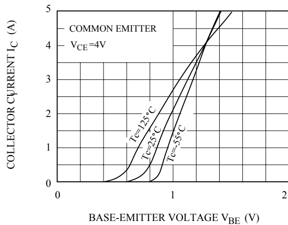
I_C - V_{BE}
