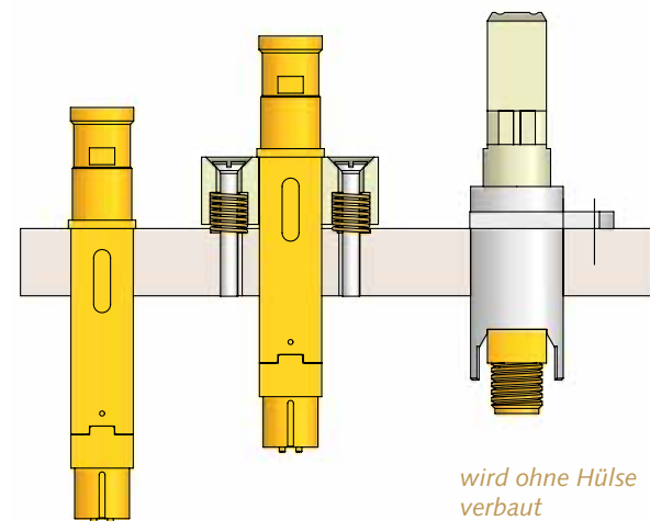
HFS ohne Kontakt- steckhülse
