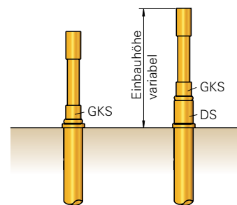
Einsatzbeispiel für KS-112 ... G8 (mit Pressring)
