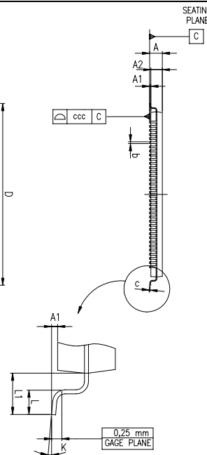
TQFP144 (20x20x1.40mm)
