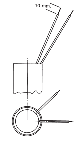
Fig. 7 Cavetti unipolari 0,5mm 2 L = 150 mm
