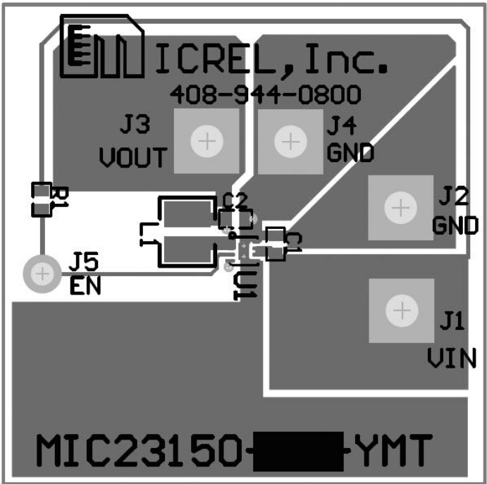
Top Layer
