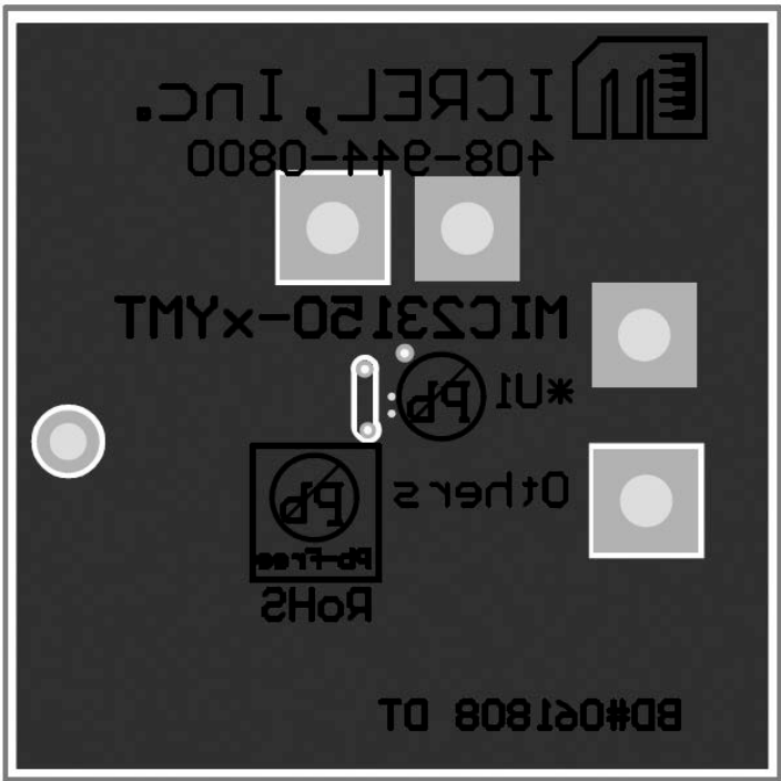
Bottom Layer
