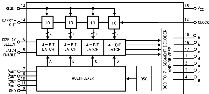
MM74C926
