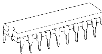
DIP20-P-300-2.54A
