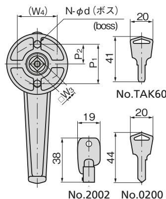
キーNo.0200 Key
