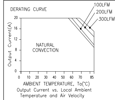
SRDB-20E12H (Vin=8 V)
