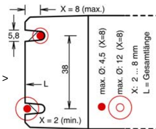
Befestigungs-Maße
